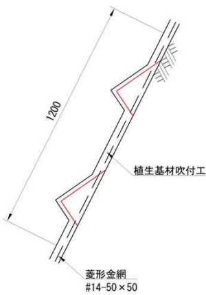
平吹付施工図
