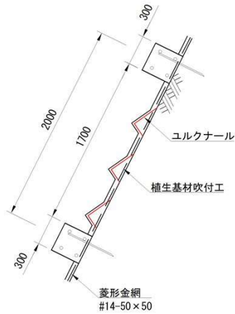
吹付のり枠内施工図
